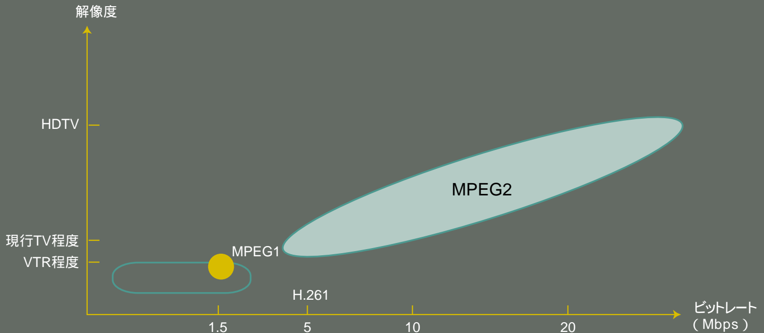
MPEG-2がカバーする伝送速度と画面解像度 MPEG-2 coverage of transmission speeds and screen resolutions
