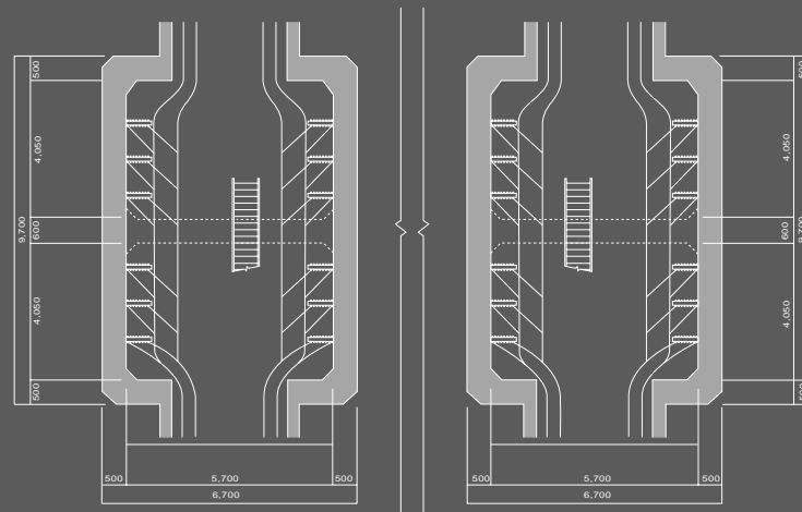
平断面図
