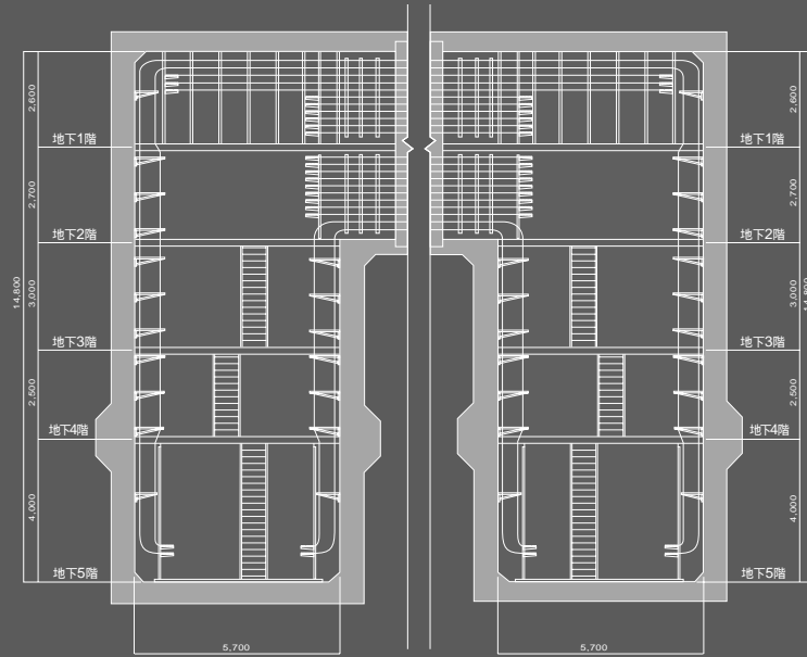
立断面図
