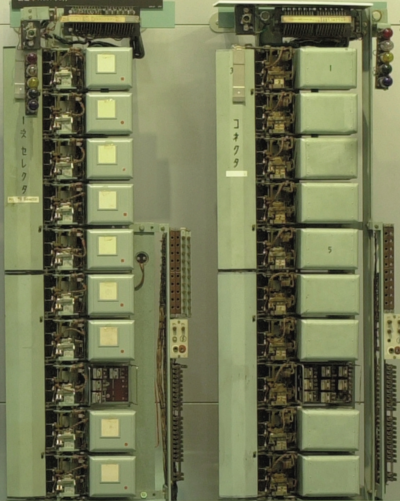
H型交換機 セレクタ架 SXS H Type Selector Frame 製造年：1951年8月
