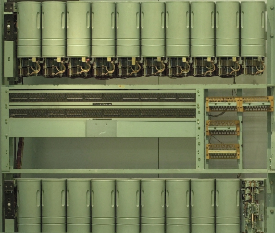
A型交換機 セレクタ架 SXS A Type Selector Frame 製造年：1955年9月
